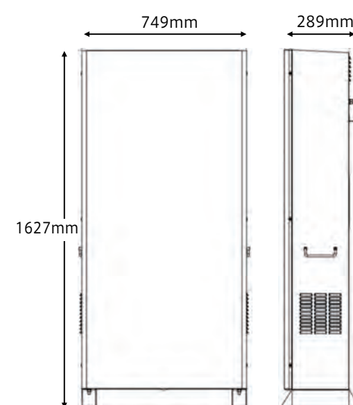
外装ケース J1ESS-HB58 J1ESS-HB115/173
