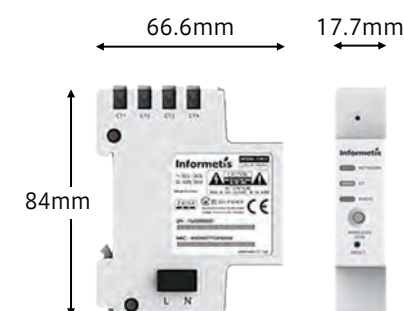
サーキットメータ CM-2/J
