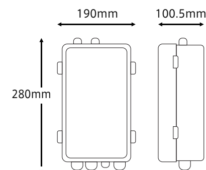
通信ユニット EJ-HGW002K
